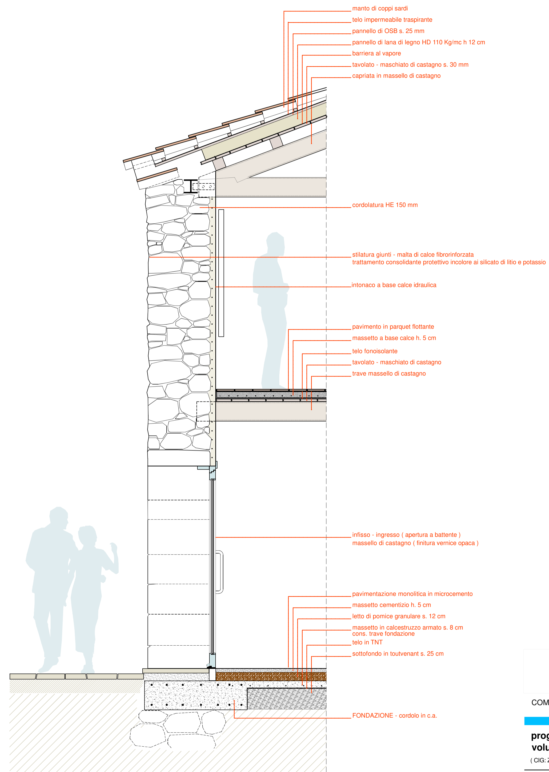
PARTICOLARI sezione tipo [ corpo B ]
