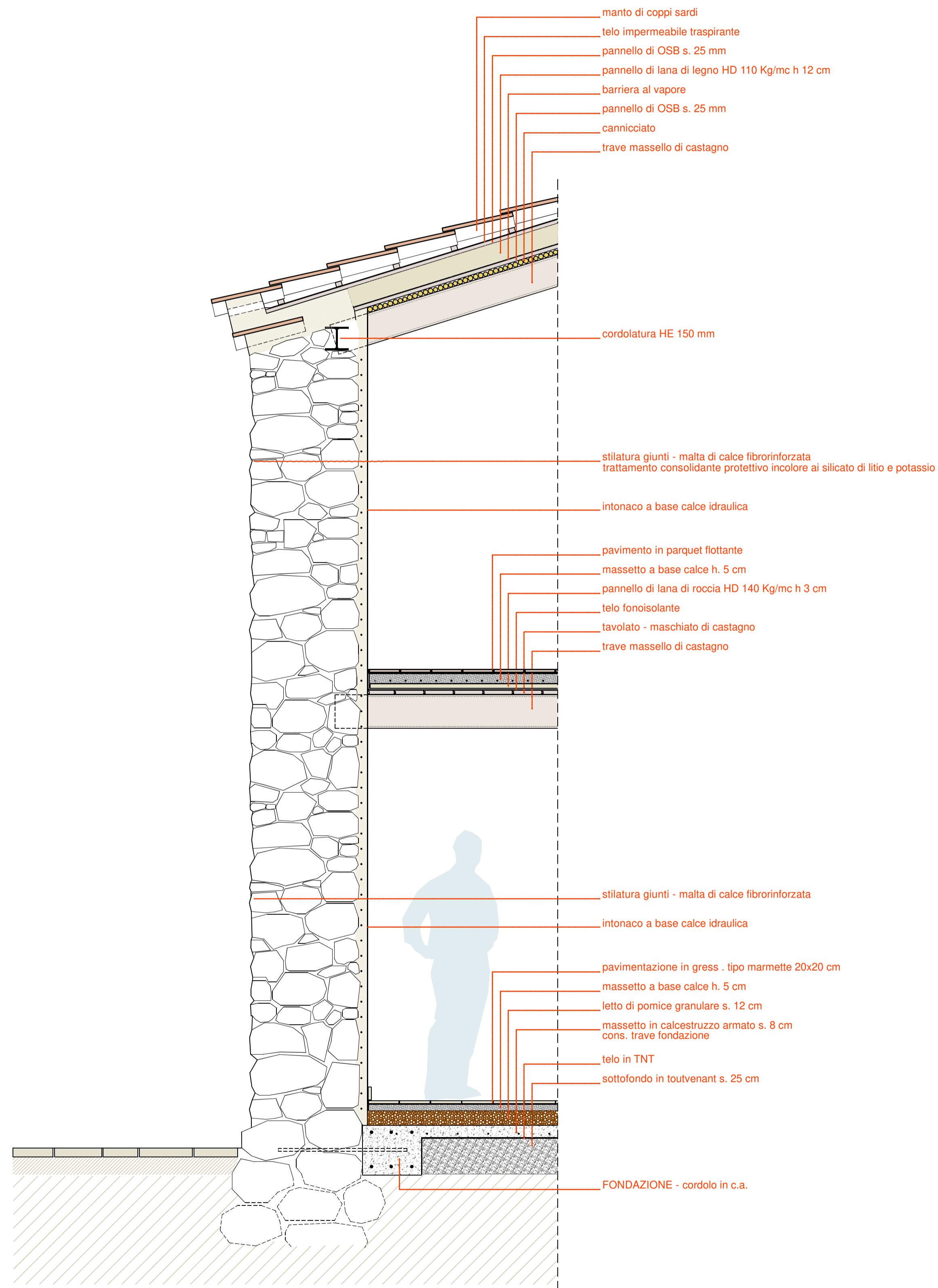
PARTICOLARI sezione tipo [ corpo A ]
